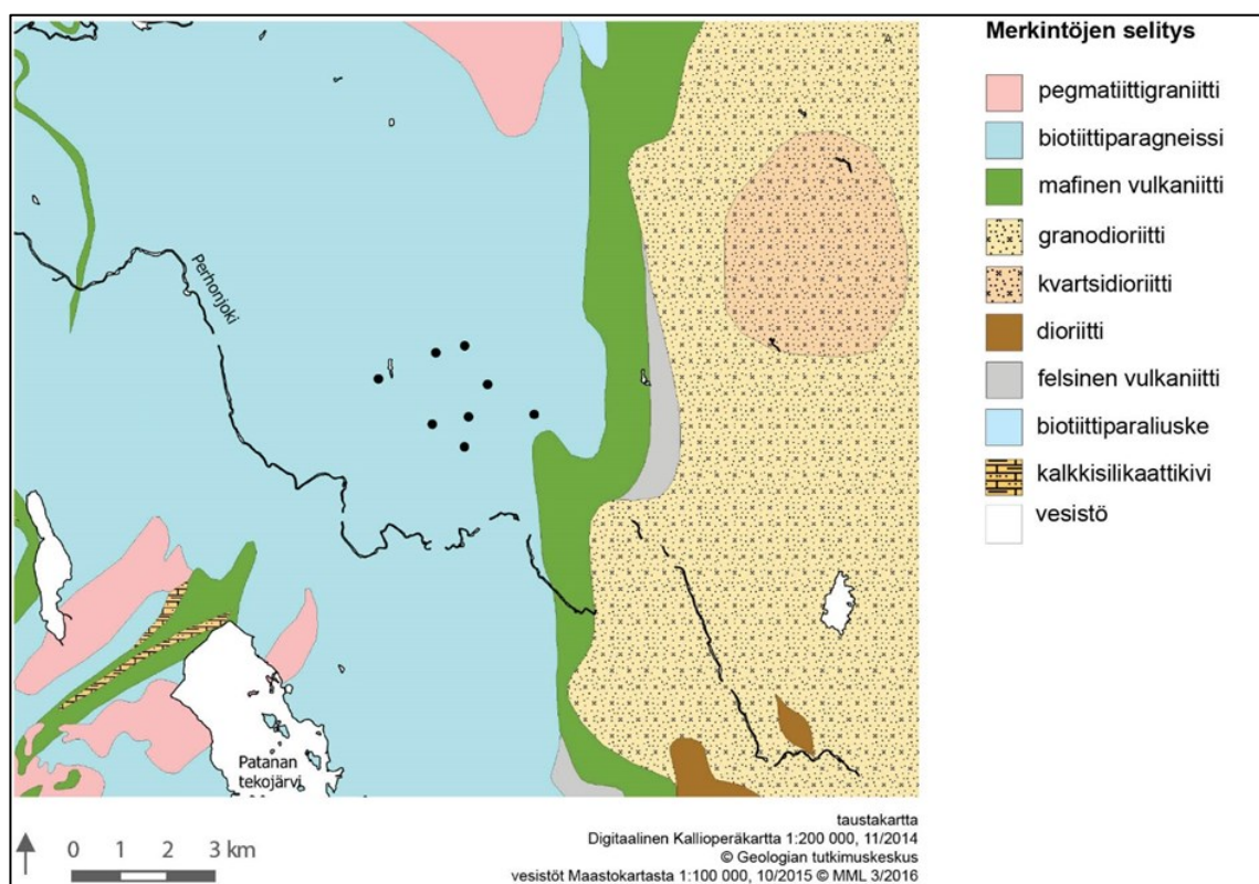
Kuva 20. Kaava-alueen kallioperäkarta.
