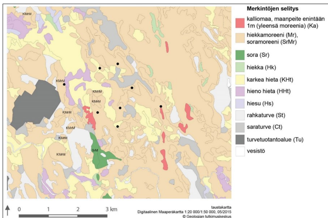
Kuva 21. Kaava-alueen maaperäkarta
