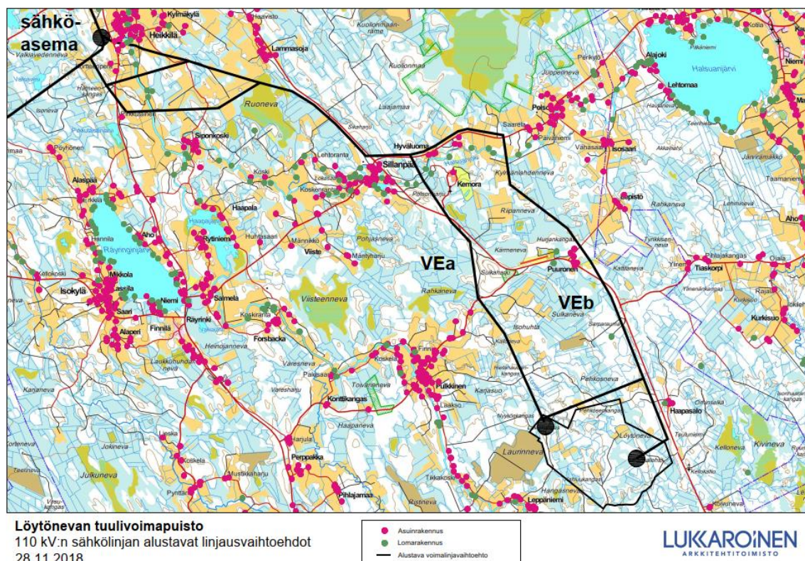
Kuva 40. Kuva 2. Löytönevan tuulivoimahankkeen alustavat 110 kV sähkönsiirtoreittivaihtoehdot.
